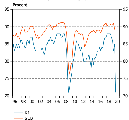
Diagram 1: Kapacitetsutnyttjande i tillverkningsind.
