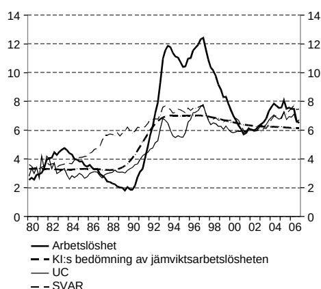
Diagram 19 Arbetslöshet Procent
