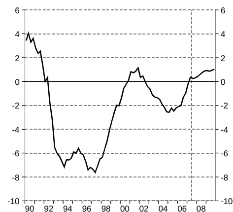
Diagram 1 Arbetsmarknadsgap
