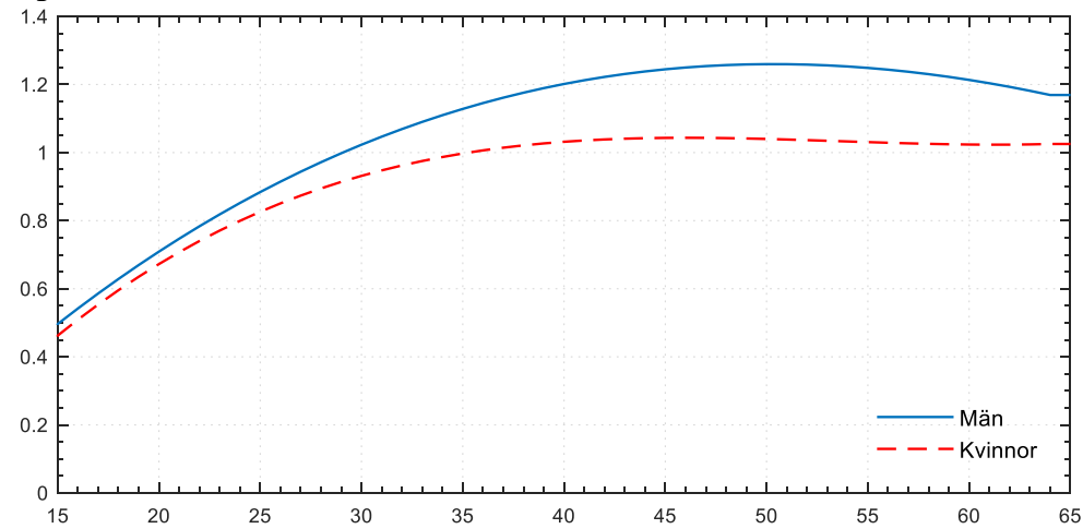
Figur 3.1: Ålderseffektivitet
