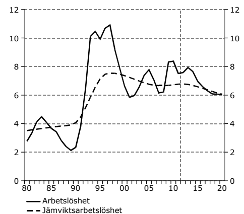
Diagram 135 Arbetslöshet
