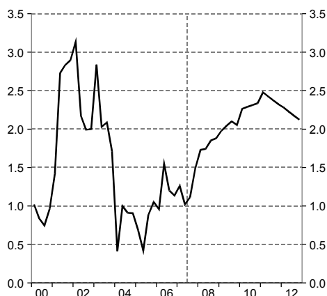
Diagram 73 UND1X-inflationen med prognostiserad reporäntebana
